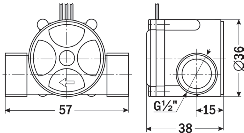
Рис. 3 – Размеры прибора
